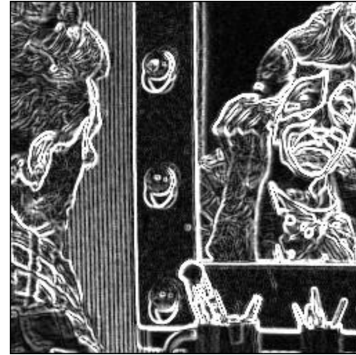
Sobel
